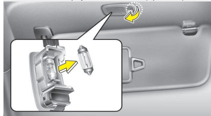
Luces de los espejos de cortesia (opcional)
